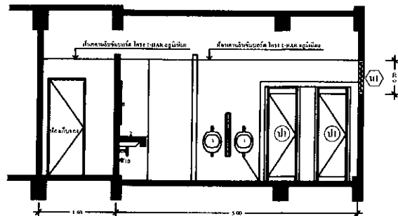
รูปตัด 1
