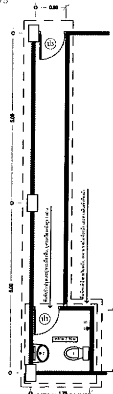
แปลนห้องน้ำ ① ชั้น G ประตูเบี่ยง
