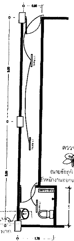
แปลนไฟฟ้าห้องน้ำ ① ชั้น G มาตราส่วน 1:75
