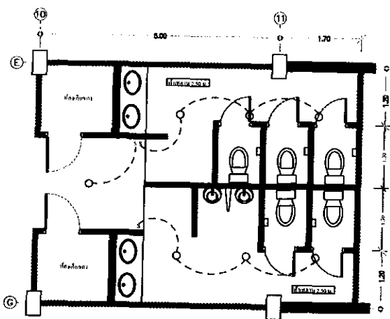
แปลนไฟฟ้าห้องน้ำรวม ② ชั้น 1, 2, 3, 4 มาตราส่วน 1:75
