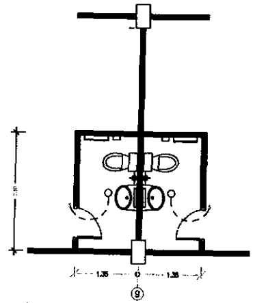
แปลนไฟฟ้าห้องน้ำ ③ ชั้น 1 (ในห้อง 109 และห้อง 111) มาตราส่วน 1:75
