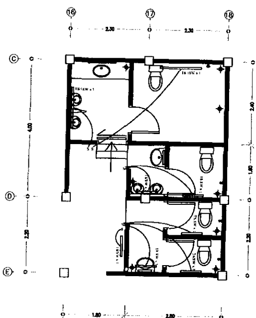
แปลนไฟฟ้าห้องน้ำ ④ มาตราส่วน 1:75
