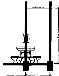
รูปตัด 3
