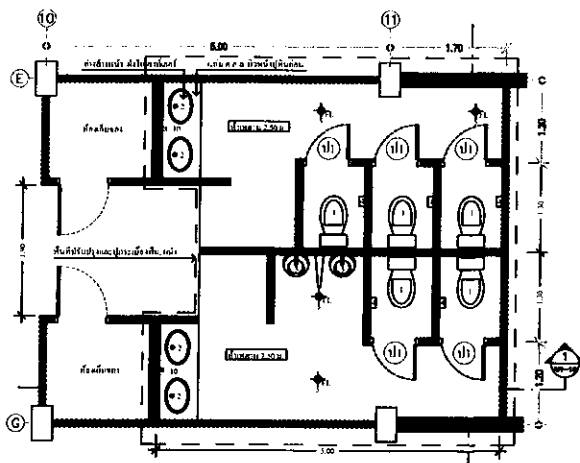
แปลนปรับปรุงห้องน้ำรวม ② ชั้น 1, 2, 3, 4
