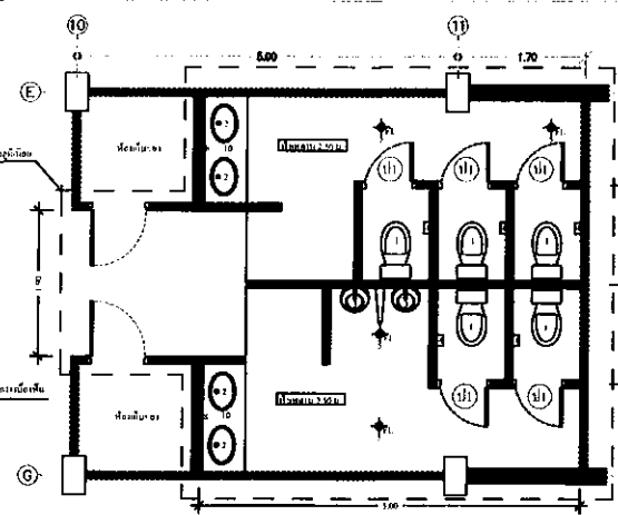
แปลนพื้นที่ปรับปรุงลิฟต์และทาสีห้องน้ำรวม ② ชั้น 1, 2, 3, 4
