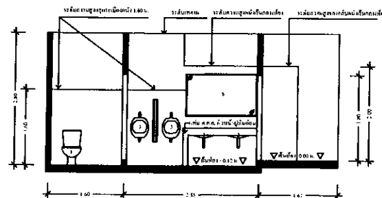
รูปตัด 6 มาตราส่วน 1:75
