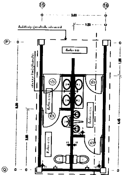
แปลนห้องน้ำ ⑤ มาตราส่วน 1:75
