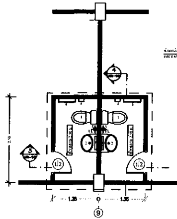
แปลนห้องน้ำ ③ ชั้น 1 (ในห้อง 109 และห้อง 111)
