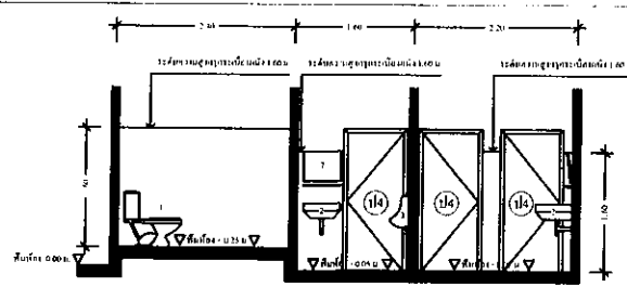
รูปตัด 5 มาตราส่วน 1:75
