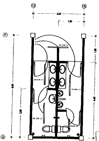
แปลนไฟฟ้าห้องน้ำ ⑤ มาตราส่วน 1:75
