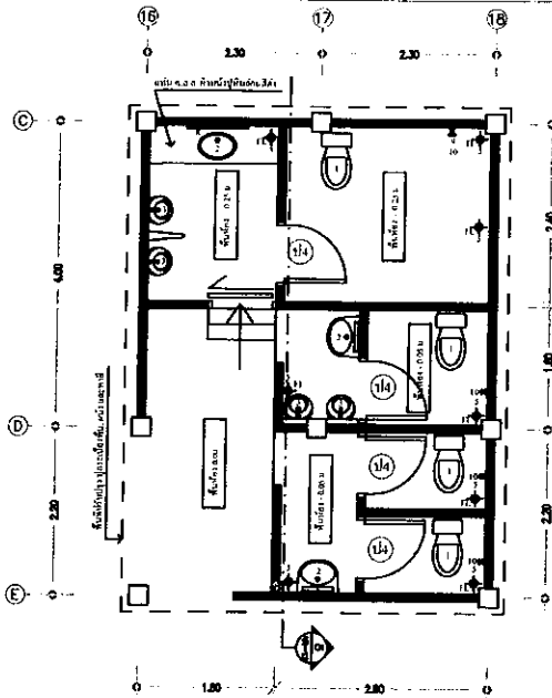
แปลนห้องน้ำ ④ มาตราส่วน 1:75
